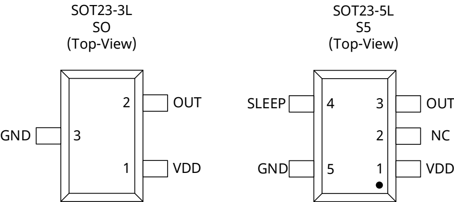
图 2. SOT23-3L 封装俯视图(左) & SOT23-5L 封装俯视图(右)
