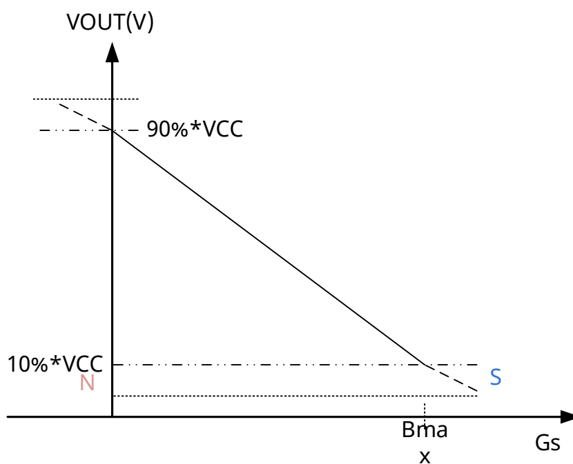
图 8. 输出函数
