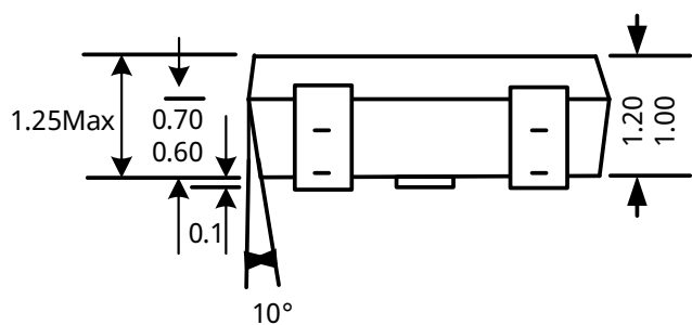
3-脚 SOT23-3L 封装
