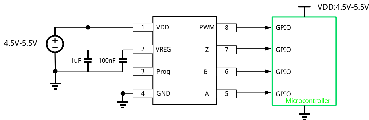
典型应用图
