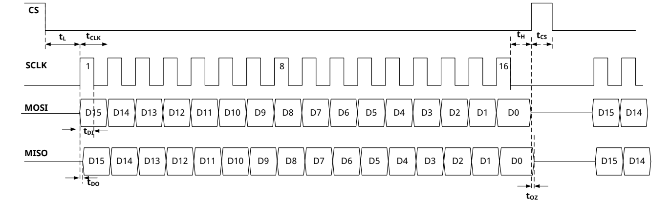
图 8 SPI 寄存器读写模式图
