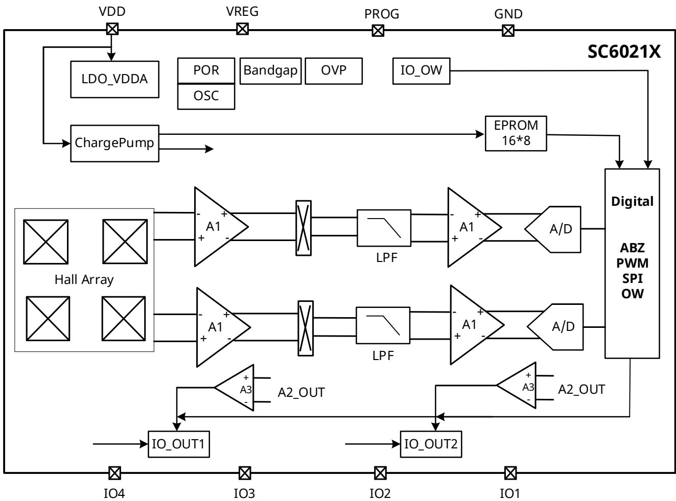
图 3 功能框图
