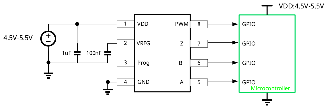
典型应用图
