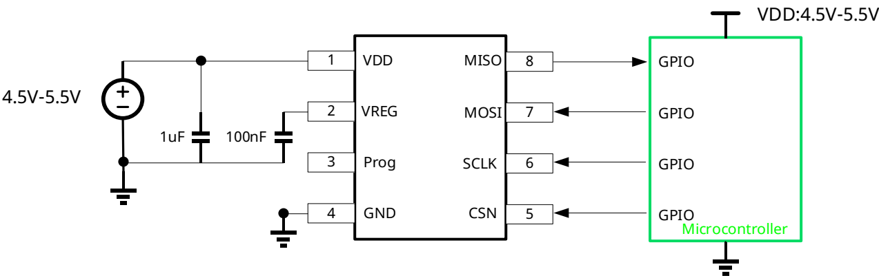
典型应用图
