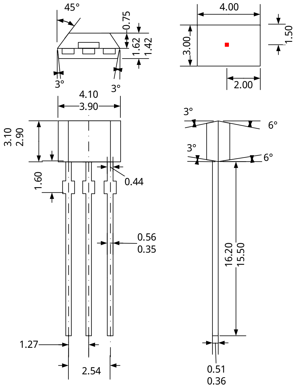
TO-92S PKG
