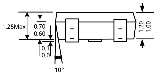
3-脚 SOT23-3L 封装
