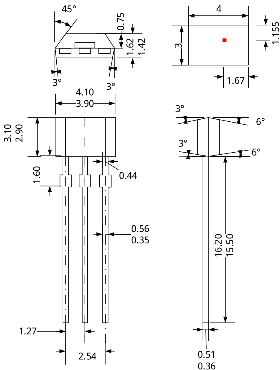
UA 封装
