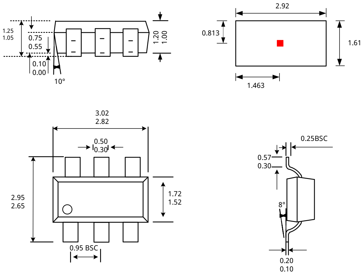
6-脚 S6 封装
