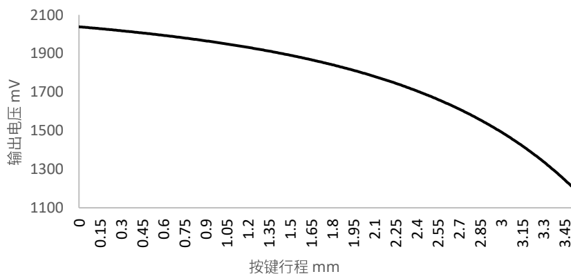
图 5. SOT23-3L 封装形式输出曲线
