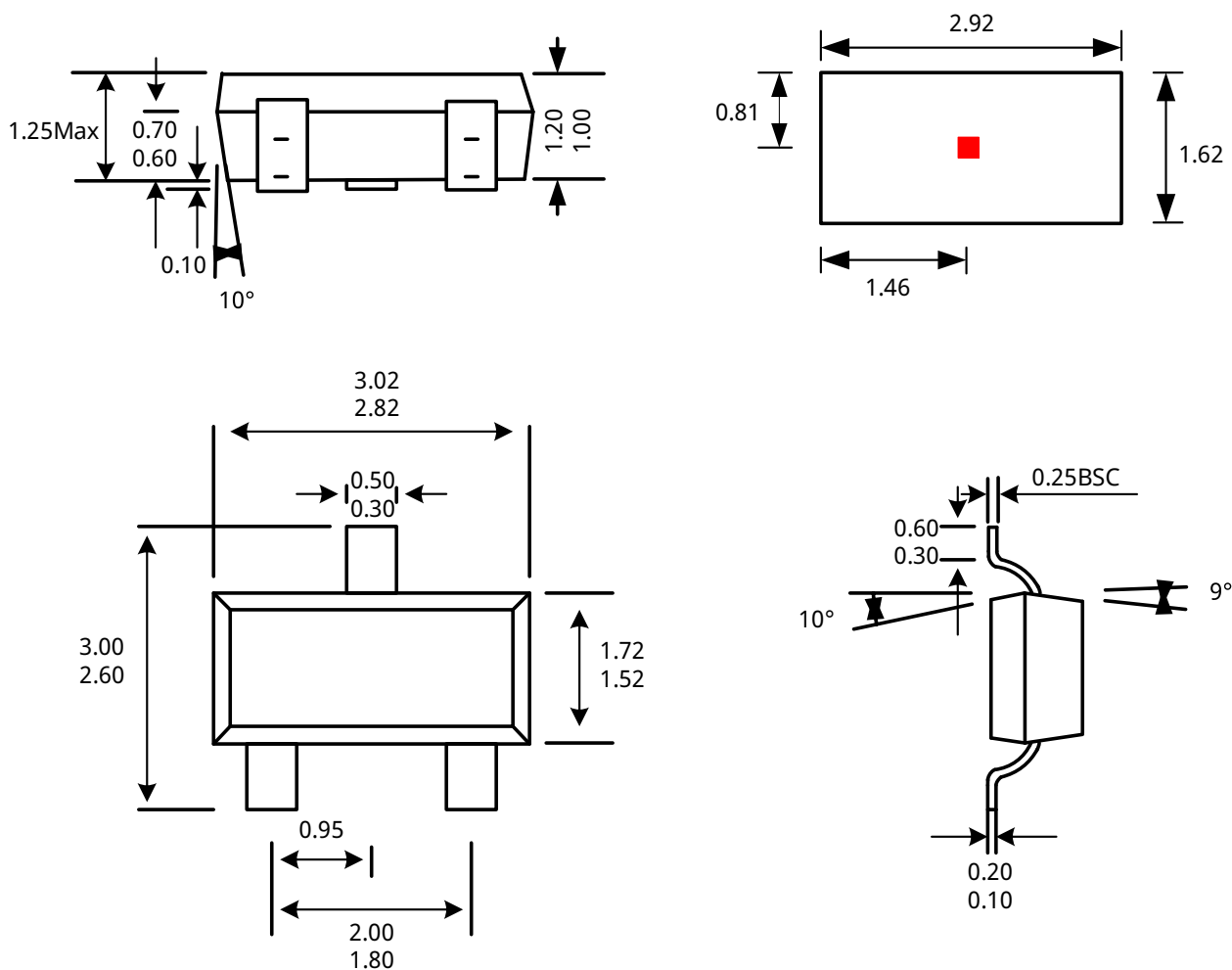
3-脚 SOT23-3L 封装
