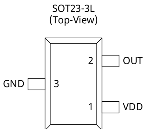
图 2. SOT23-3L 封装俯视图
