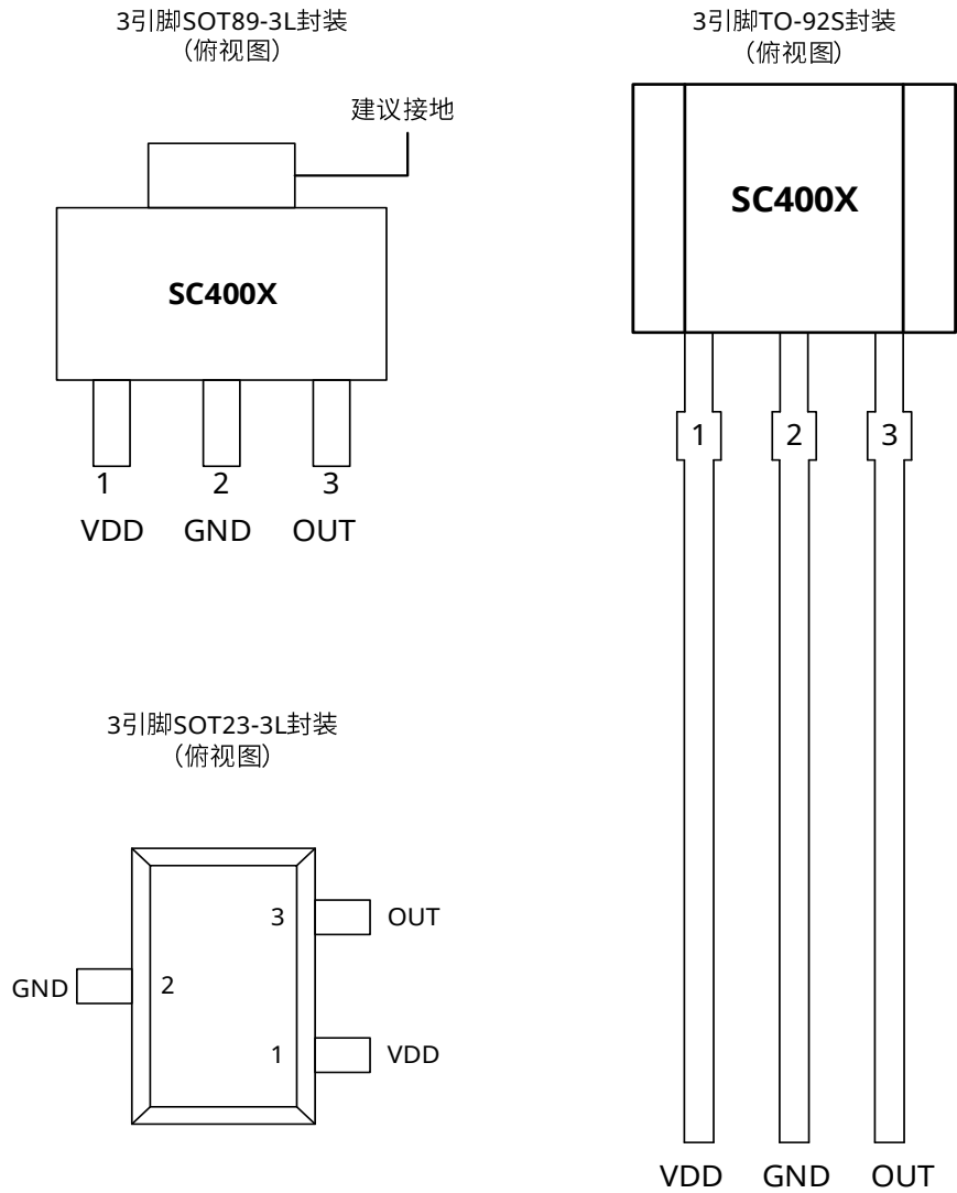
图 2. SOT89-3L 封装俯视图(左上) & SOT23-3L 封装俯视图(左下) & TO-92S 封装俯视图(右)
